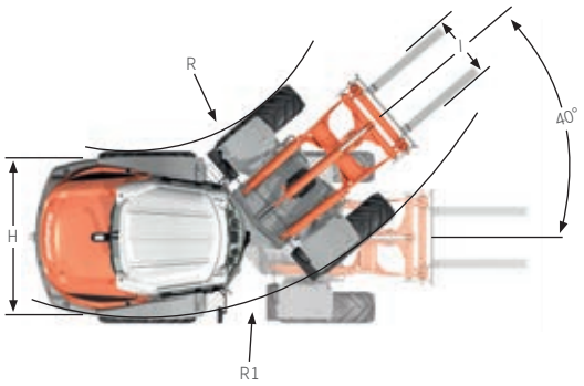
Mit Palettengabel
