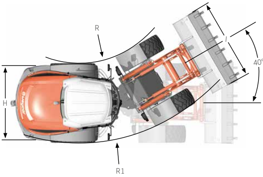
Mit Standardschaufel
