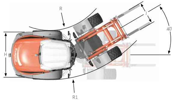
Mit Palettengabel
