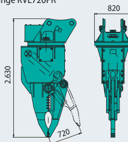
Multi-Demontage- zange KVE720PR
