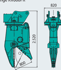
Fahrzeug-Demontage- zange KV800PR
