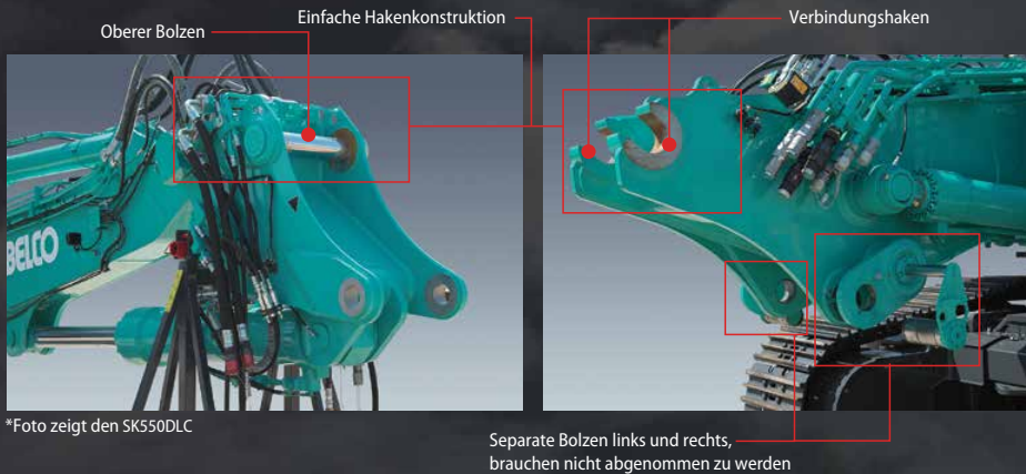
Separate Bolzen links und rechts Führung
