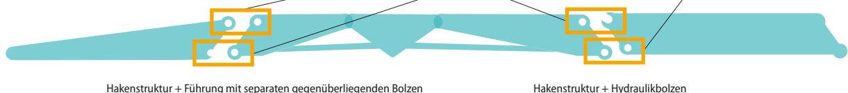
Hakenstruktur + Führung mit separaten gegenüberliegenden Bolzen
