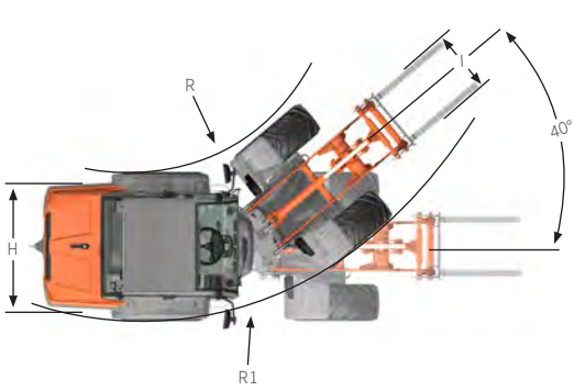
Mit Palettengabel
