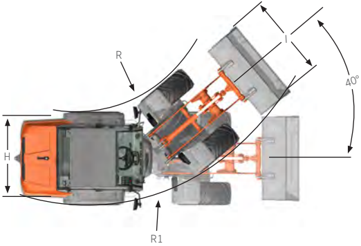
Mit Standardschaufel
