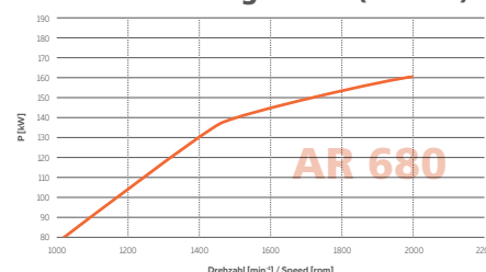
Motorleistungskurve (AR 680)
